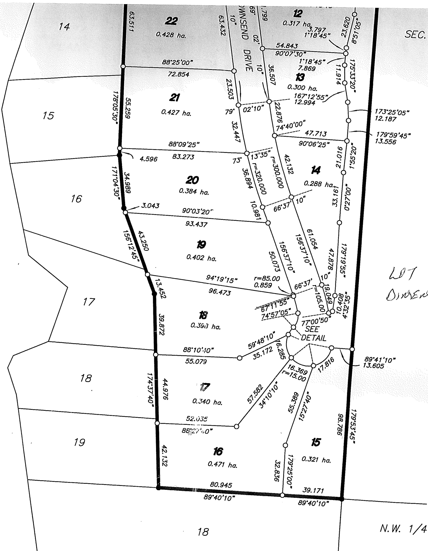
PLAN 27209
