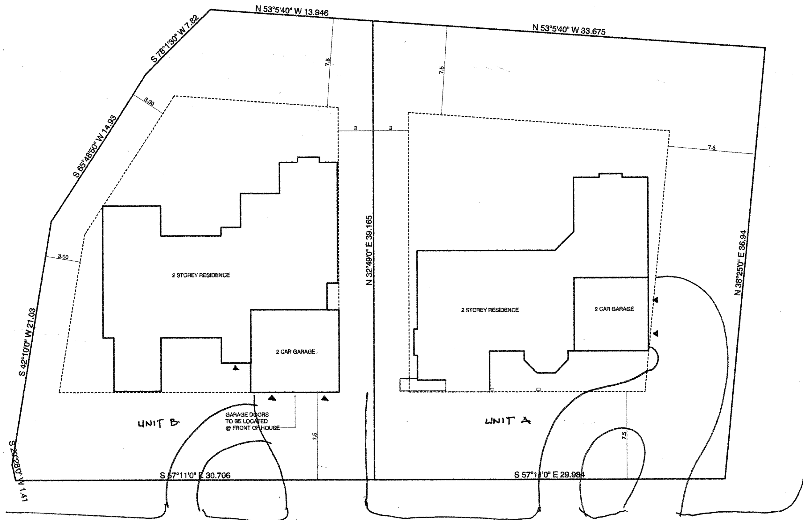
SITE PLAN (OPTION B) SCALE: 1: 200
