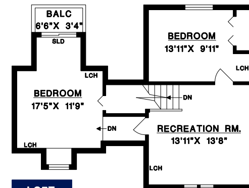
LOFT
